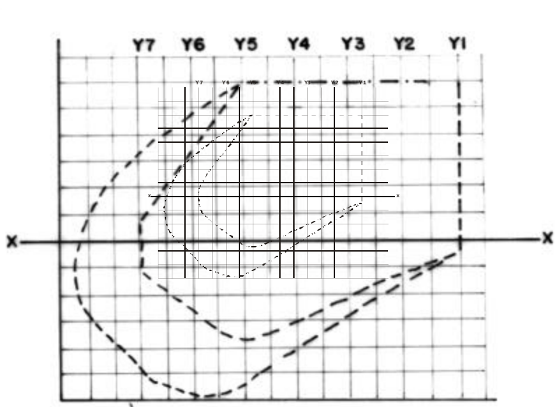
Figura E.1 Levantamiento de un terreno con cinta métrica
