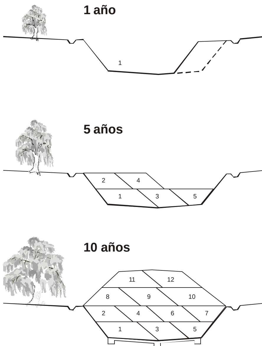
Figura 7.9 Secuencia de la construcción de terraplenes para el llenado del terreno
