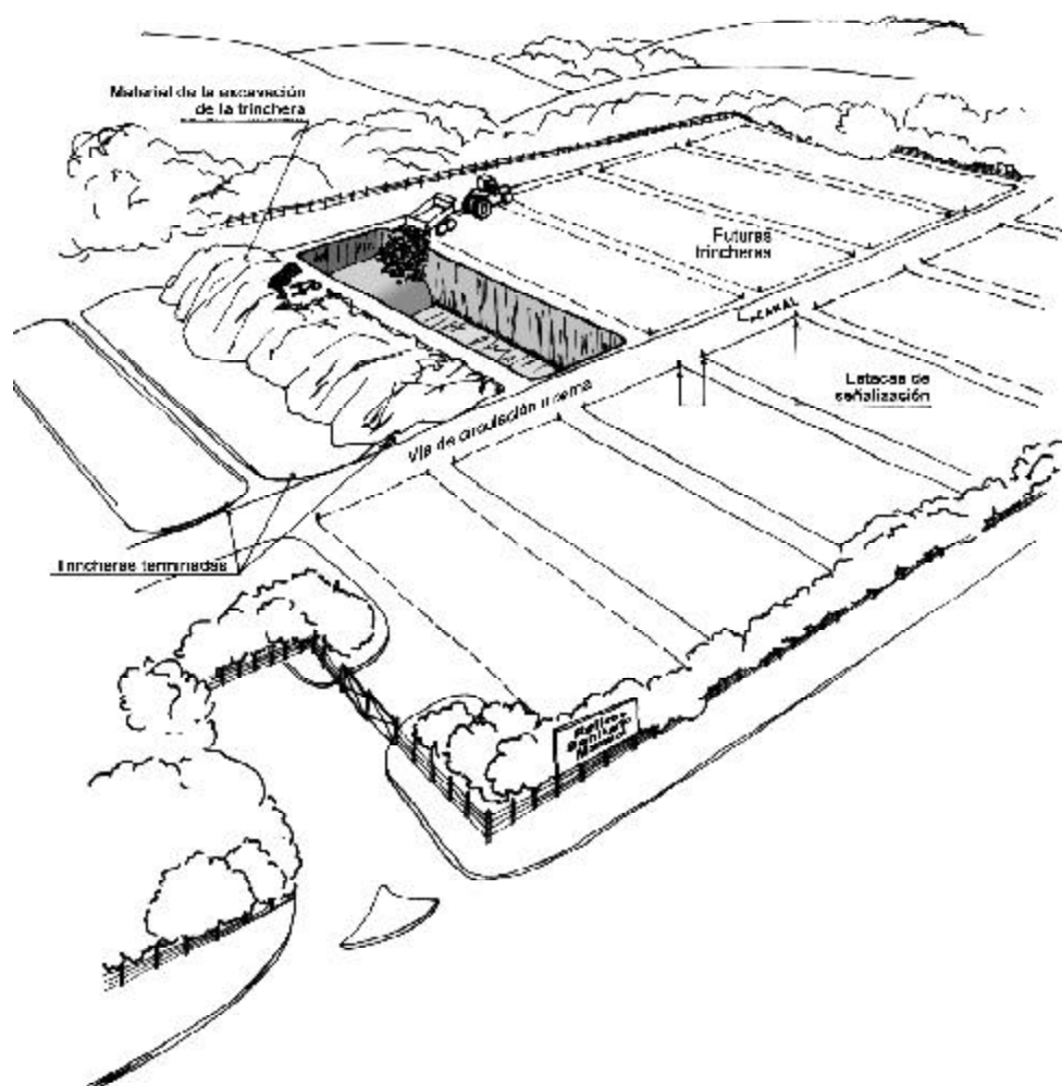
Figura 7.7 Plan de manejo del terreno para la construcción del relleno sanitario manual mediante el método de trinchera
