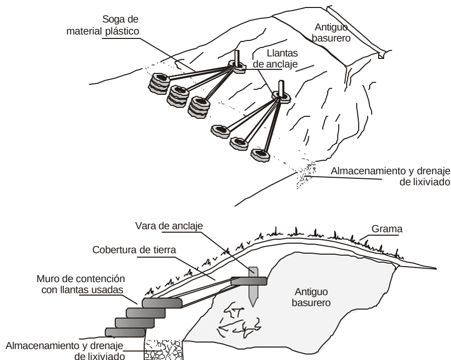
Figura 9.4 Controles para la estabilidad de taludes con llantas de automotores
