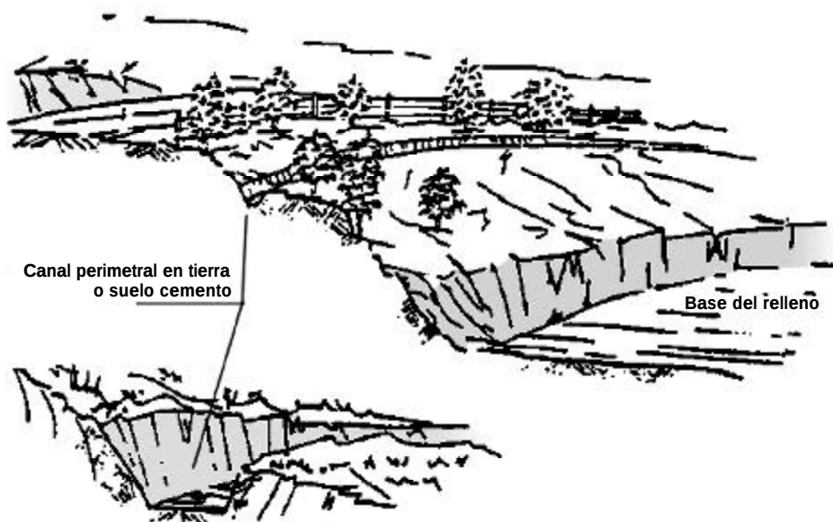
Figura 5.14 Drenaje perimetral para desviar las aguas de lluvia y red para lixiviado
