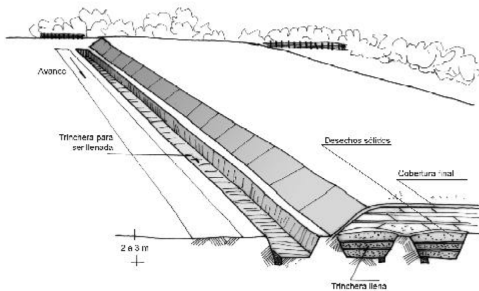
Figura 3.8 Combinación de ambos métodos para construir un relleno sanitario
