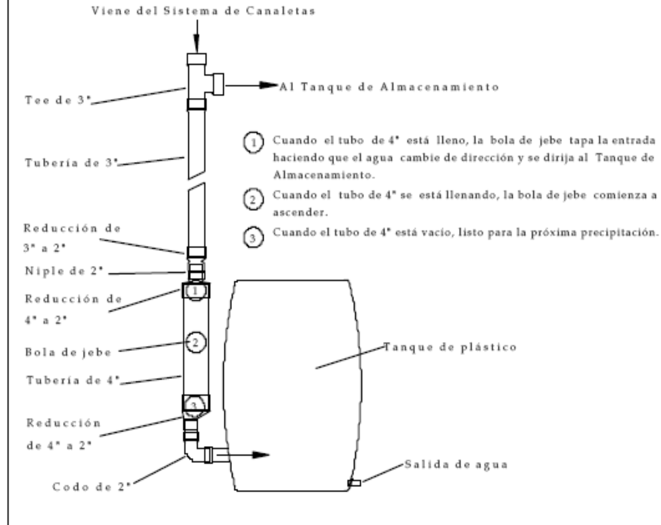
Figura 3. Interceptor de Primeras Aguas
